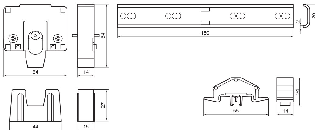
Механизм блокировки
